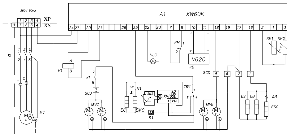
Рис.1. (трехфазное питание)
