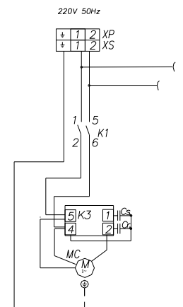
Рис.2. (однофазное питание) остальное см. рис.1
