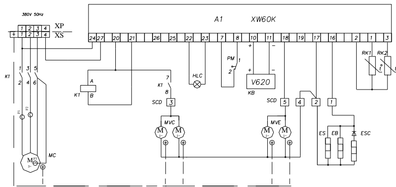
Рис.1. (трехфазное питание)
