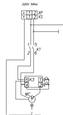
Рис.2. (однофазное питание) остальное см. рис.1
