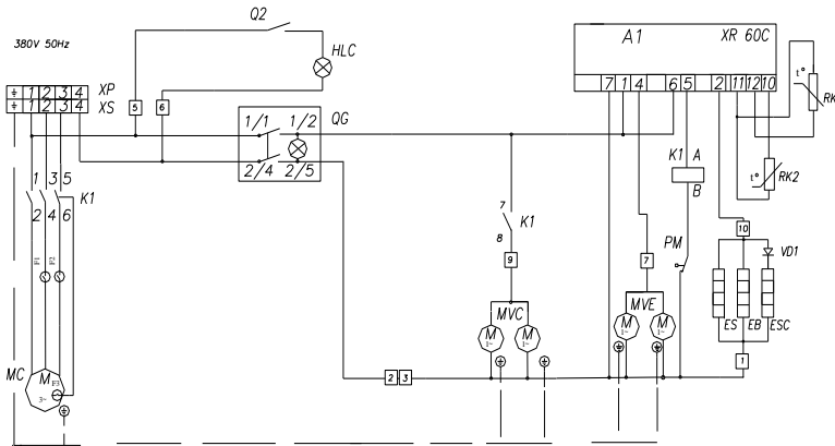
Рис.1 (трехфазное питание)
